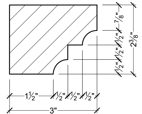
B TRIM SECTION SCALE: 1/2" = 1"
