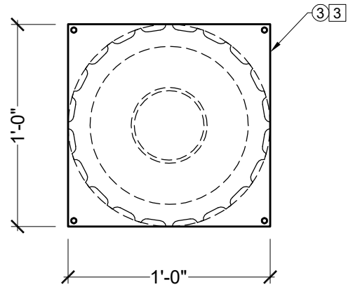
TOP VIEW SCALE: 1/8" = 1"
