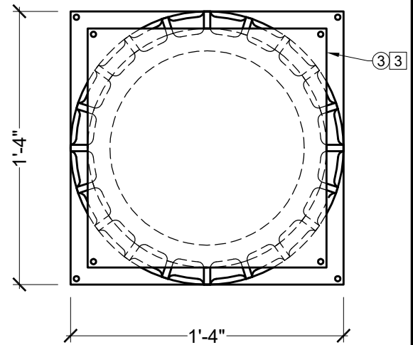
TOP VIEW SCALE: \frac{1}{8}'' = 1''
