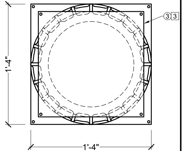
TOP VIEW SCALE: 3/8" = 1"
