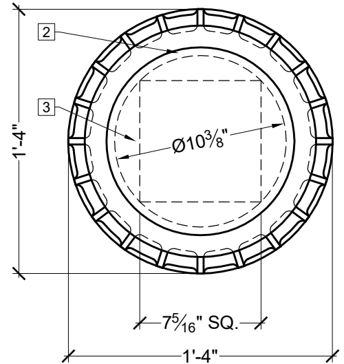
TOP VIEW SCALE: 3/8" = 1"
